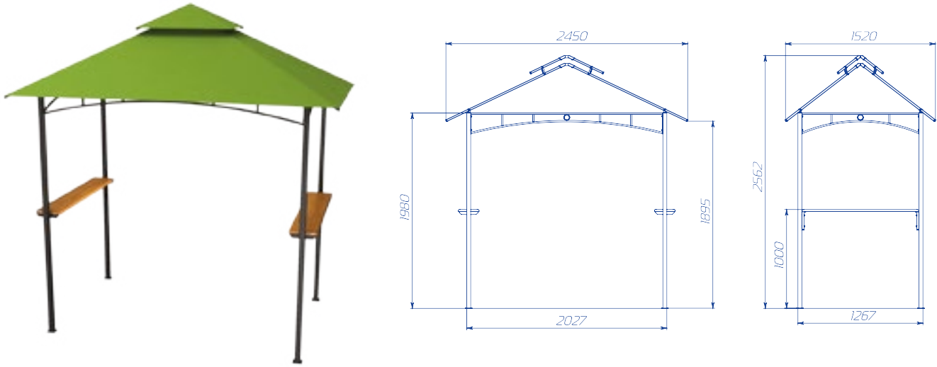
HOLIDAY TENT 3X3 НАМЕТ ДЛЯ ВІДПОЧИНКУ 3X3
