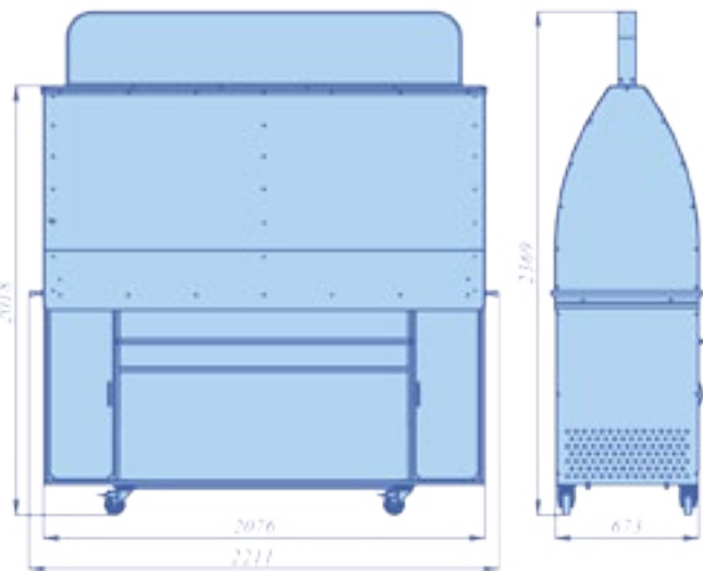
Chest freezer trolley Візок під морозильну скриню
