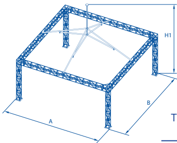
PAVILION DOMICAL, REINFORCED ПАВІЛЬЙОН КУПОЛЬНИЙ, ПОСИЛЕНИЙ
